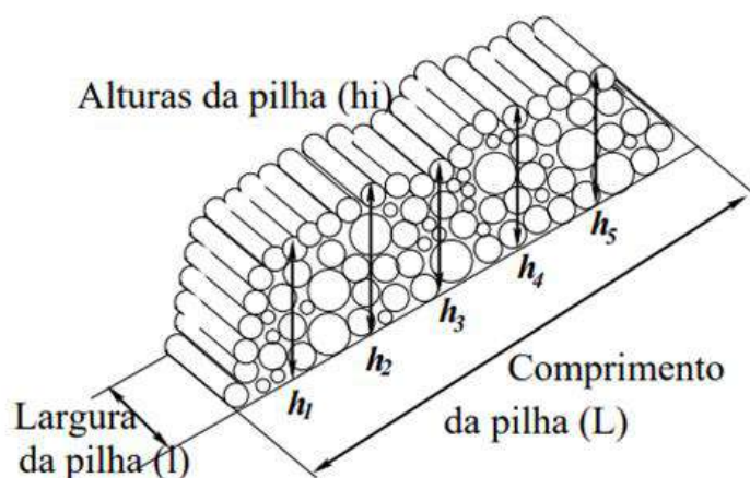
Figura 1.7.2. Representação da pilha de lenha.
