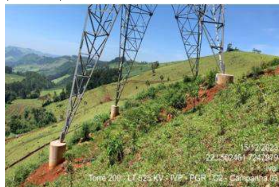
Figura 1.3.13. Dispositivos de drenagem à montante das bases de ancoragem inferiores, funcionais (Torre 200).
