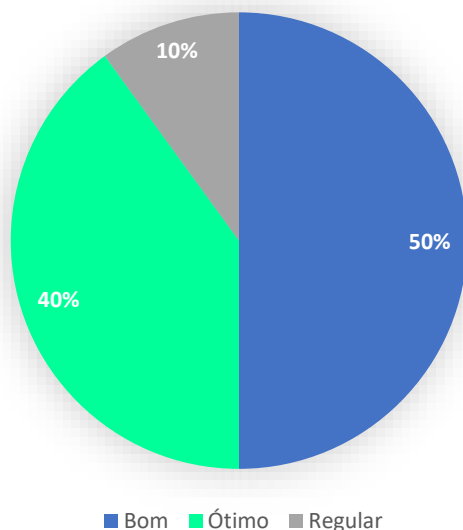
Figura 1.3.22. Status das áreas em recuperação ambiental.
